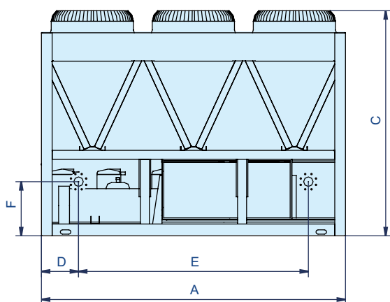
Вид спереди
