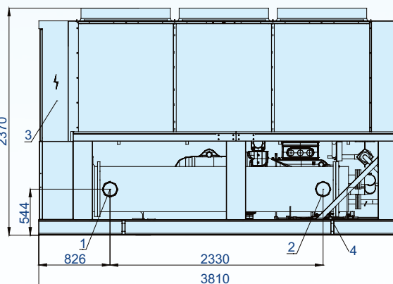
ВИД СПЕРЕДИ
