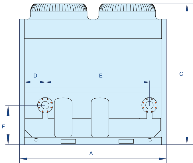
Вид спереди
