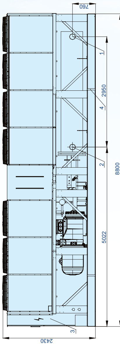
ВИД СПЕРЕДИ
