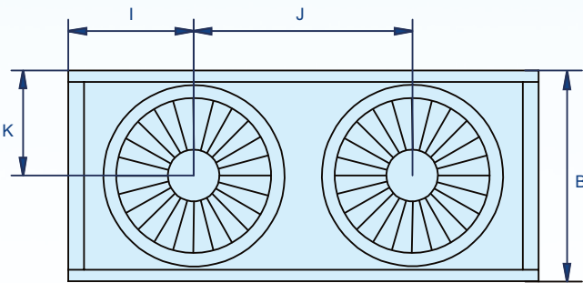
Вид сверху
