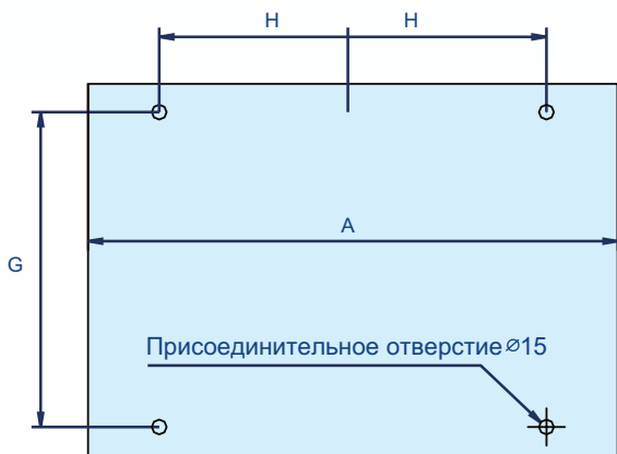
Присоединительные отверстия
