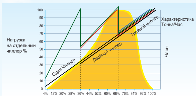
Пример рабочих характеристик трёх чиллеров
