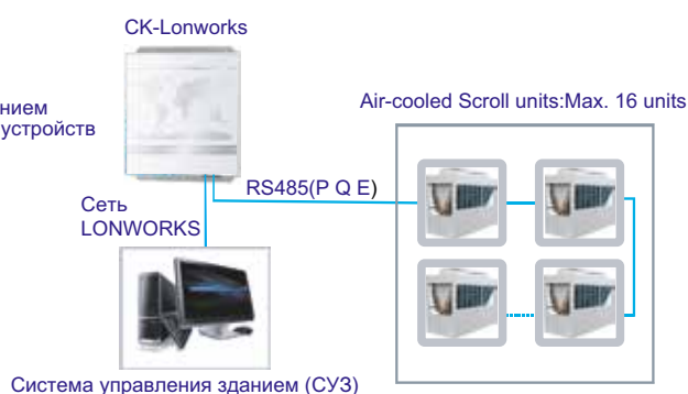
Способ подключения 2
