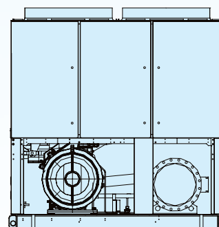
ВИД СБОКУ
