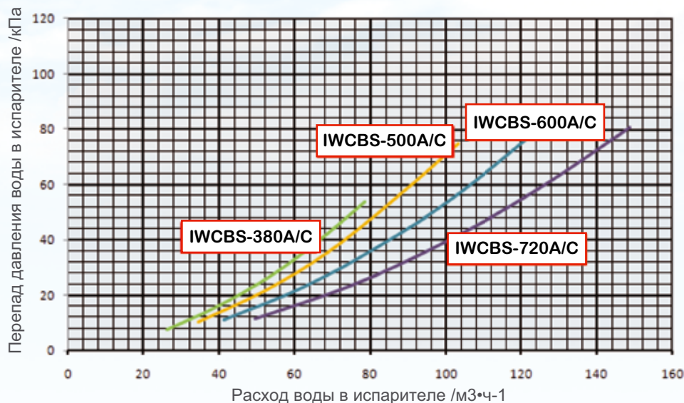
Характеристика перепада давления воды в испарителе
