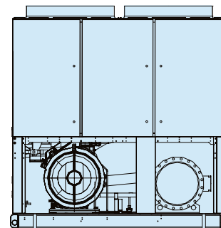
ВИД СБОКУ
