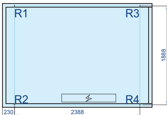
Модуль 200 кВт
