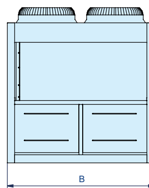
Вид слева
