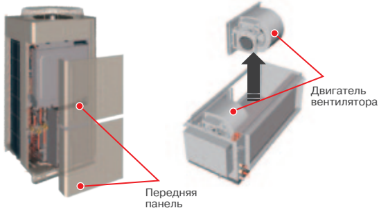
Наружный блок
