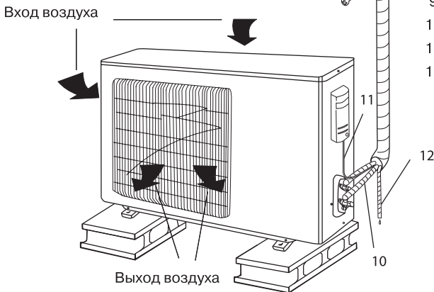
Наружный блок
