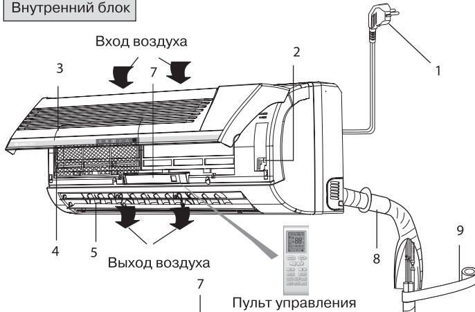
Внутренний блок
