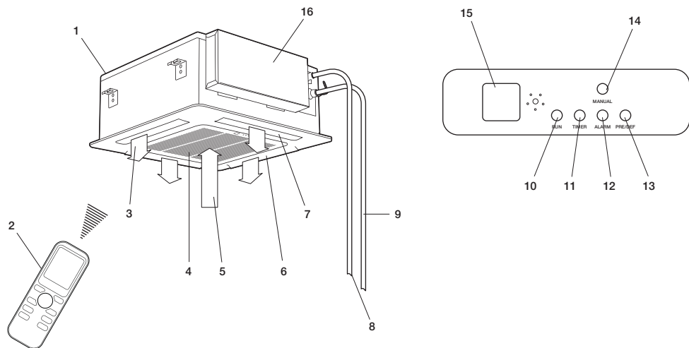
Рис. 1. Устройство внутреннего блока: 1 — внутренний блок; 2 — беспроводной пульт дистанционного управления; 3 — выход воздуха; 4 — воздухозаборная решетка с воздушным фильтром; 5 — вход воздуха; 6 — воздуховыпускная решетка; 7 — направляющая заслонка; 8 — соединительные трубопроводы; 9 — шланг для отвода конденсата; 10 — индикатор работы; 11 — индикатор работы по таймеру; 12 — индикатор аварийного состояния; 13 — индикатор режима оттаивания DEF; 14 — кнопка ручного управления; 15 — приемник инфракрасных сигналов пульта дистанционного управления; 16 — насос для отвода конденсата из внутреннего блока
